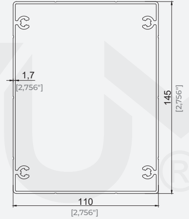
110x145 Dikme Profili 110x145 Pillar Profile
