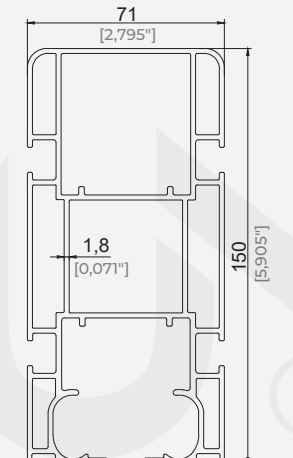
71x150 Ray Profili 71x150 Rail Profile Büküme Uygundur.
