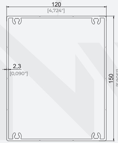
120x150 Dikme Profili 120x150 Pillar Profile
