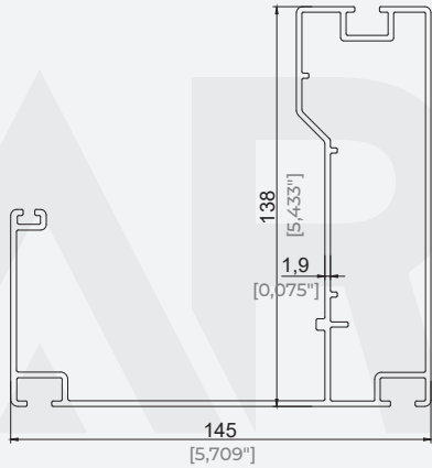
145x138 Eko Dere Profil 145x138 Eco Gutter Profile
