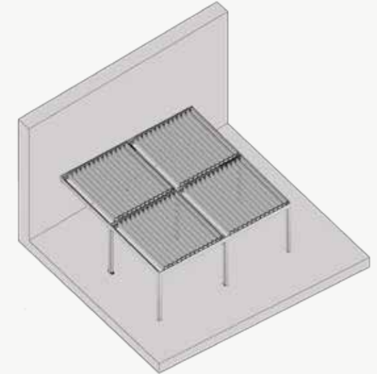
BİOKLİMATİK ÇOKLU SİSTEM VENTO MULTIPLE SYSTEM
